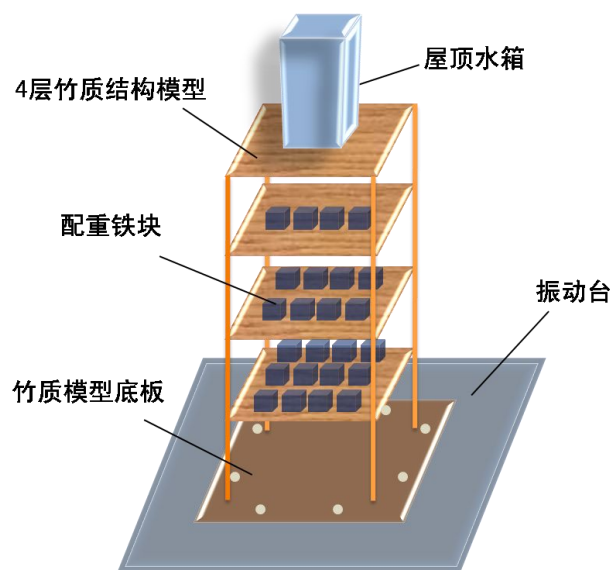
图 1 模型示意图
